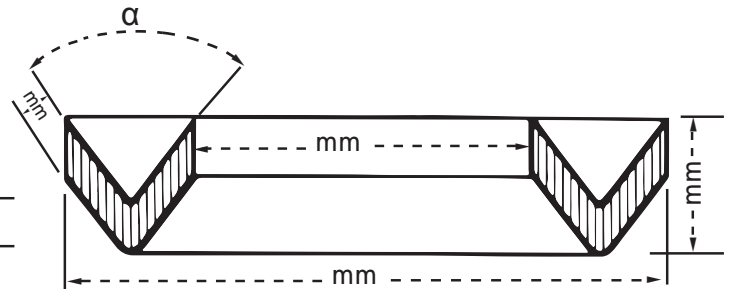
Dachform für Packungen
